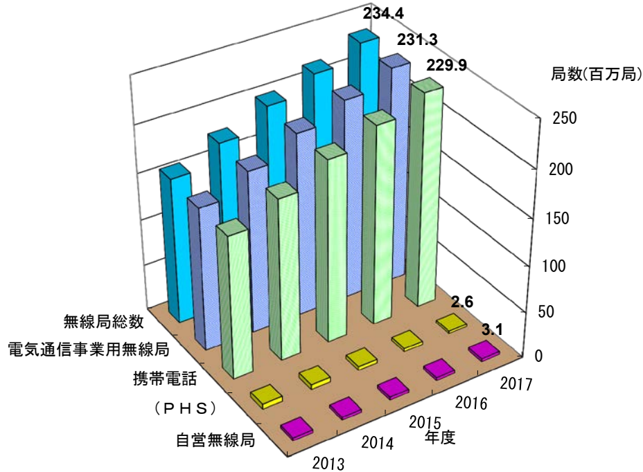
図 1-2-1 主な用途別無線局数の推移
